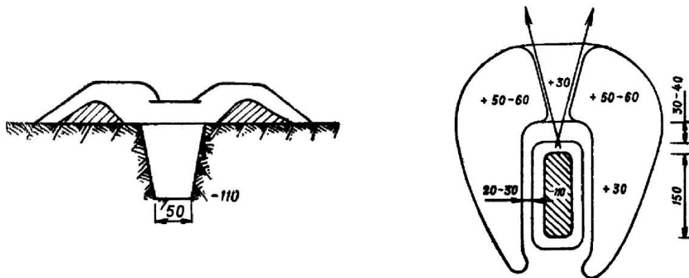
Рисунок 12. Одиночный окоп для стрельбы из автомата стоя. Вид сбоку и сверху
