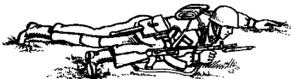
Рисунок 2. Переползание по-пластунски
