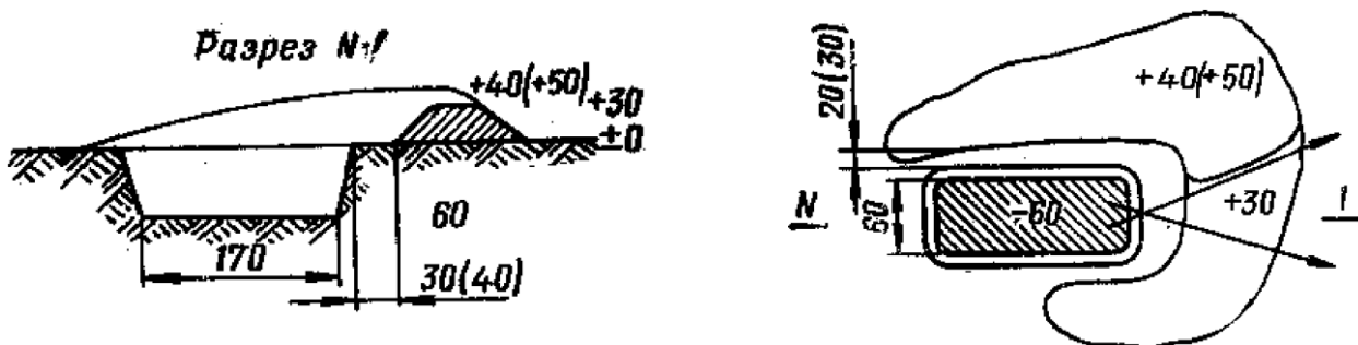
Рисунок 11. Одиночный окоп для стрельбы с колена. Вид сбоку и сверху.
