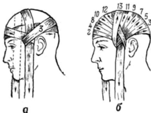
Рисунок 38. Повязка «чепец»
